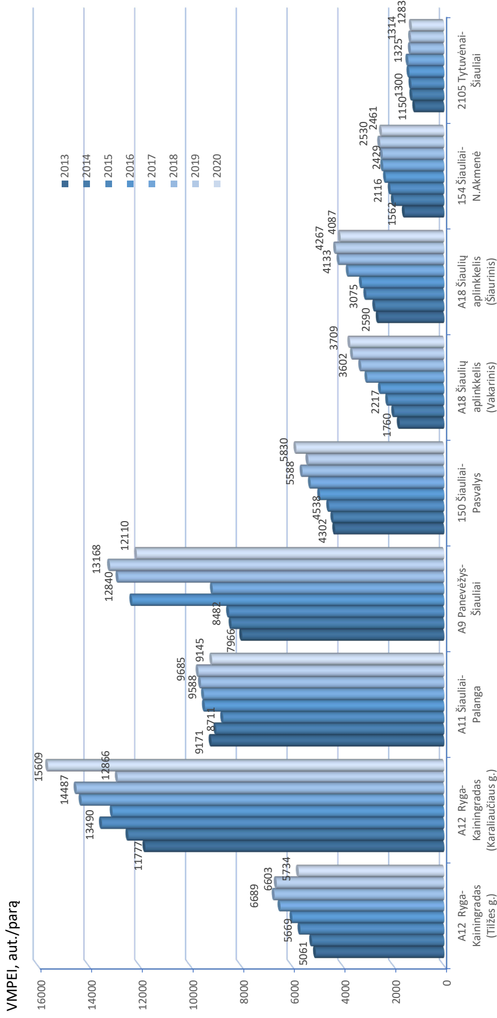
14 pav. Bendro vidutinio metinio (VMPEI) paros eismo intensyvumo kitimas magistraliniuose ir krašto keliuose Šiaulių miesto priegose 2013÷2020 m.
