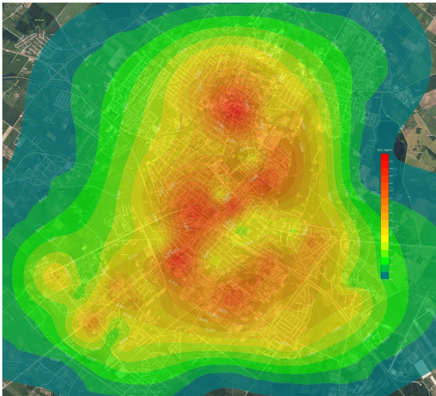
31 pav. Azoto dioksido ( \text{NO}_2 ) vidutinės valandos koncentracijos pasiskirstymas Šiaulių m. aplinkos ore 2021 m. (ribinė vertė 0,200 \text{mg/m}^3 )
