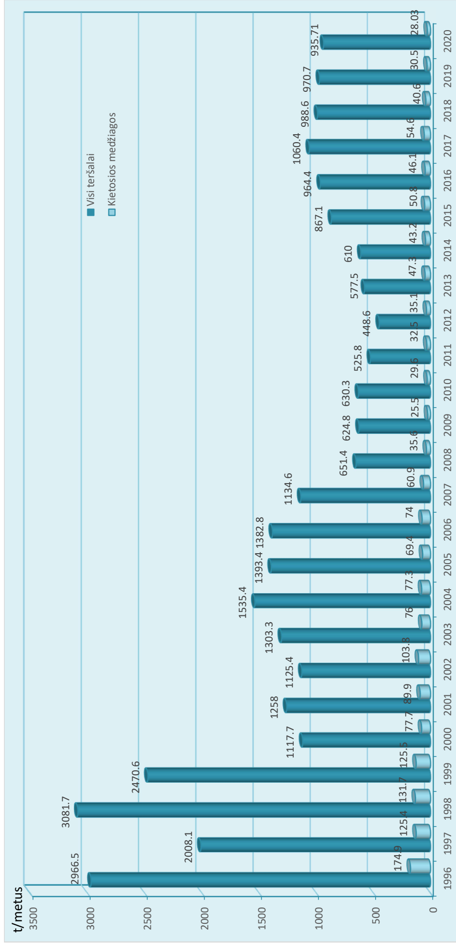
6 pav. Iš apskaitomų stacionarių aplinkos oro taršos šaltinių išmesto teršalų kiekio kitimas Šiauliuose 1996 ÷ 2020 m. laikotarpiu
