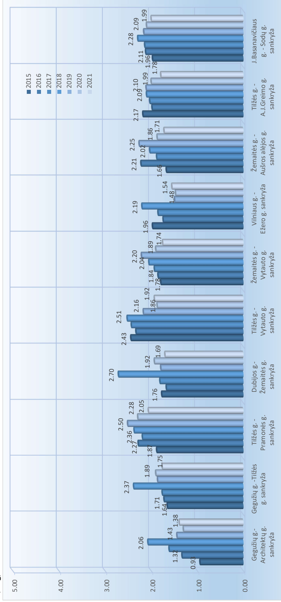
38 pav. Anglies monoksido koncentracijos kitimas pagrindinių miesto gatvių sankryžų aplinkos ore 2015÷2021 m. (Ribinė vertė gyvenamojoje aplinkoje 10 mg/m 3 )
