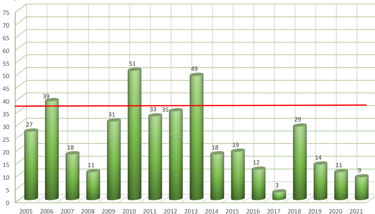
22 pav. Kietųjų dalelių (KD 10 ) vidutinės 24 val. koncentracijos viršijimų skaičiaus kitimas Šiauliuose 2005÷2021 m. (Leistinas viršijimų skaičius 35 dienos per metus)
