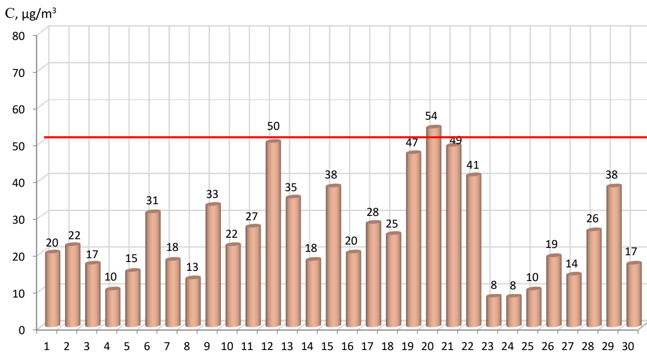
45 pav. Kietųjų dalelių ( \text{KD}_{10} ) vidutinės paros koncentracijos kitimas pietinėje miesto dalyje 2021 m. balandžio mėn. 1÷30 d.
