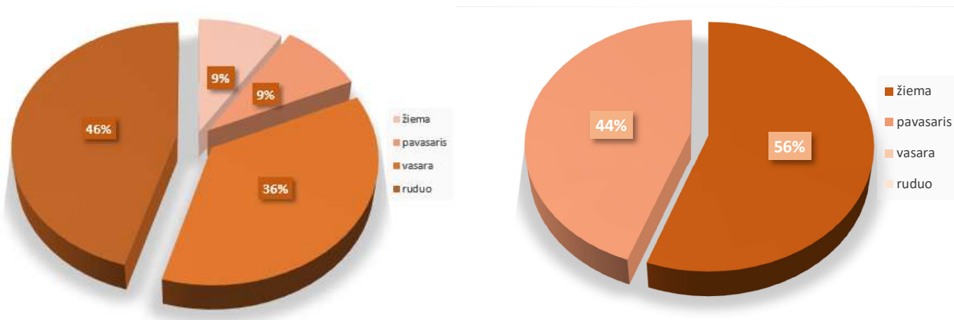
23 pav. Kietųjų dalelių ( KD_{10} ) vidutinės 24 val. koncentracijos viršijimų skaičiaus sezoninis kitimas Šiauliuose 2020, 2021 m.
