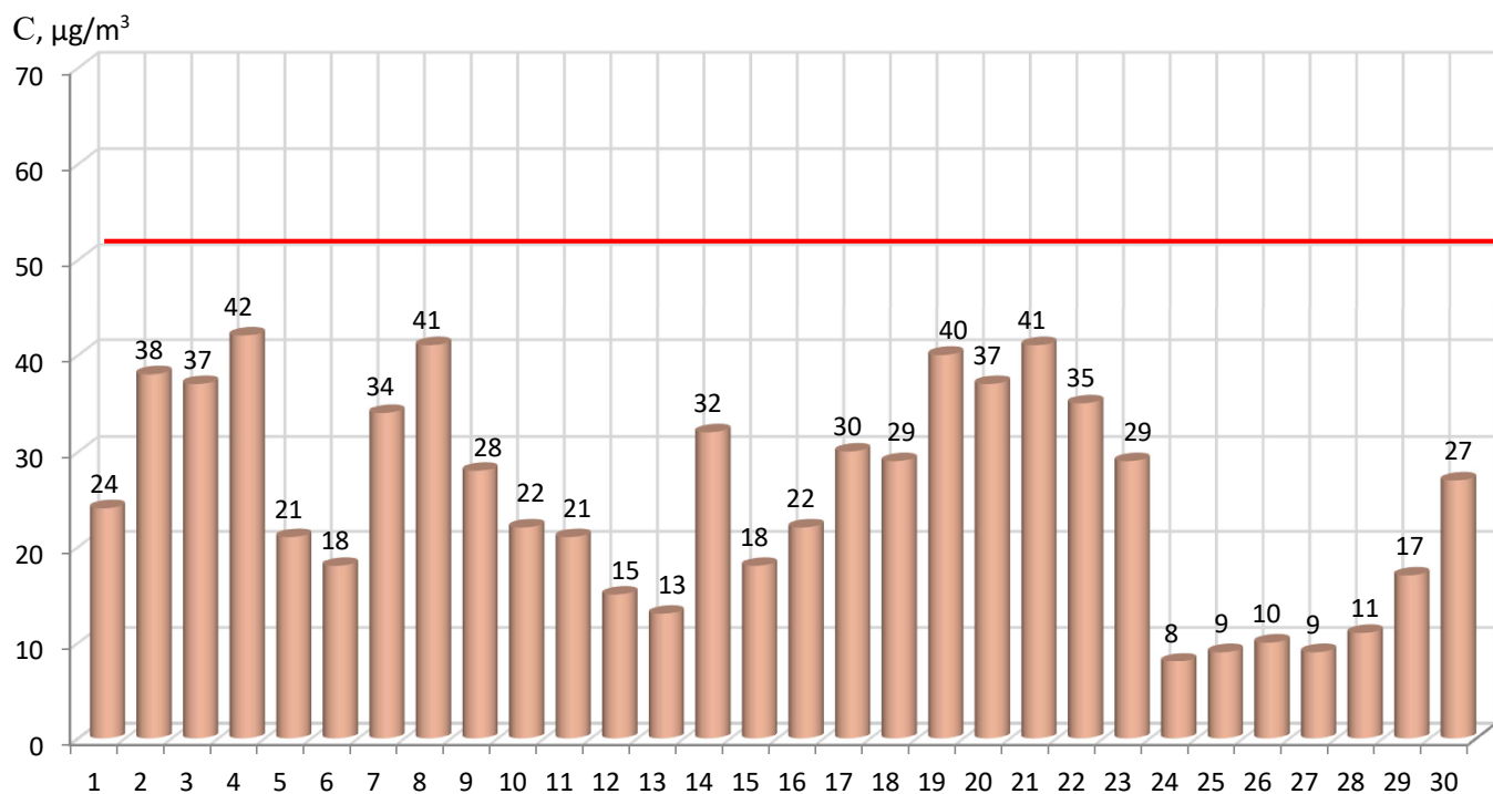
47 pav. Kietųjų dalelių ( \text{KD}_{10} ) vidutinės paros koncentracijos kitimas pietinėje miesto dalyje 2021 m. birželio mėn. 1÷30 d.
