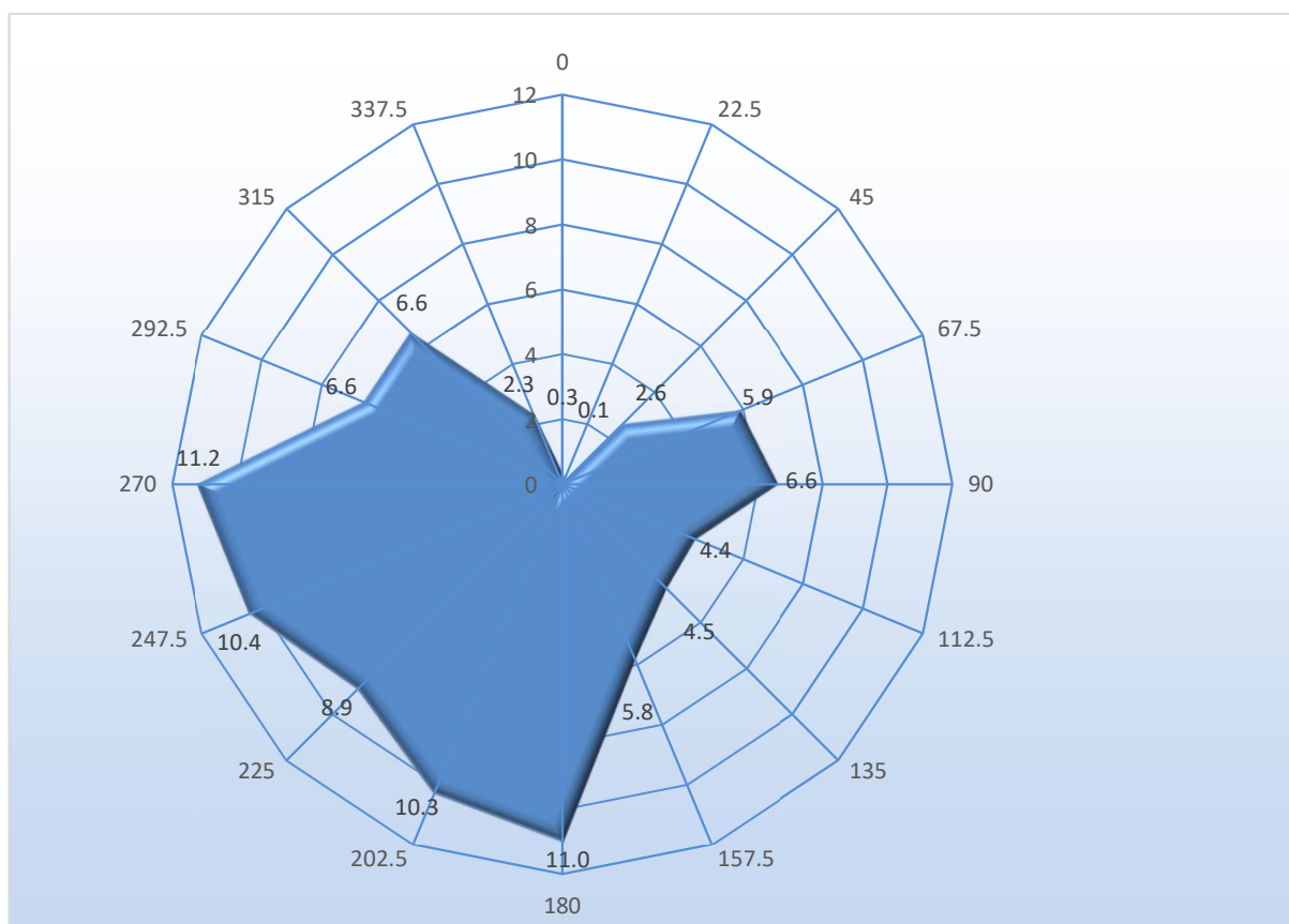
30 pav. Vyraujančių vėjo kryptių pasiskirstymas Šiauliuose 2021 m.
