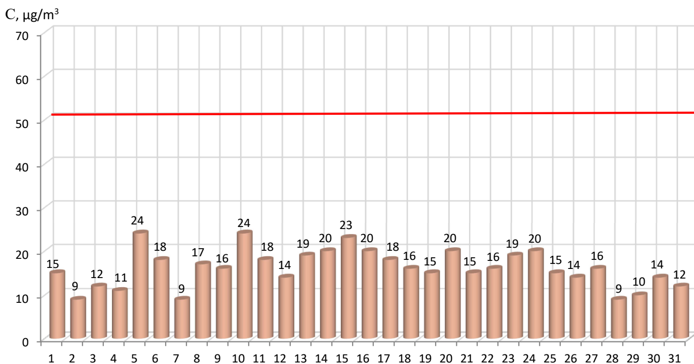
48 pav. Kietųjų dalelių ( \text{KD}_{10} ) vidutinės paros koncentracijos kitimas pietinėje miesto dalyje 2021 m. liepos mėn. 1÷31 d.
