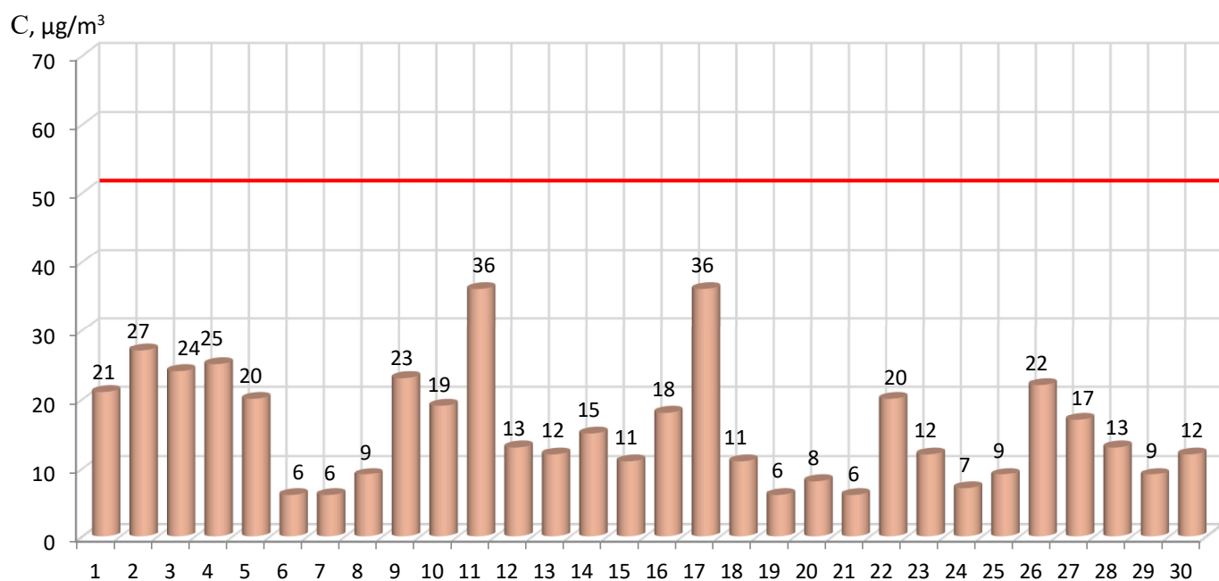
52 pav. Kietųjų dalelių ( \text{KD}_{10} ) vidutinės paros koncentracijos kitimas pietinėje miesto dalyje 2021 m. lapkričio mėn. 1÷30 d.
