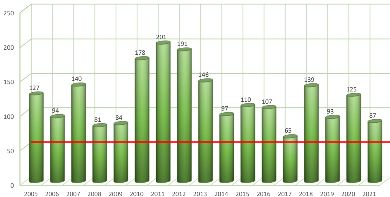
21 pav. Kietųjų dalelių (KD 10 ) maksimali 24 val. koncentracija Šiauliuose 2005÷2021 m. (Ribinė vertė 50 \mu\text{g}/\text{m}^3 )
