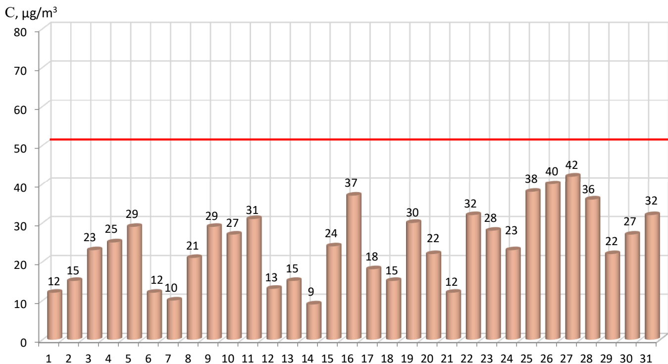
44 pav. Kietųjų dalelių ( \text{KD}_{10} ) vidutinės paros koncentracijos kitimas pietinėje miesto dalyje 2021 m. kovo mėn. 1÷31 d.
