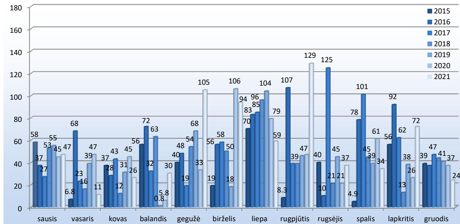
27 pav. Kritulių kiekio sezoninis kitimas Šiauliuose 2021 m.
