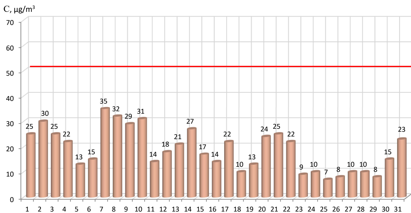
53 pav. Kietųjų dalelių ( \text{KD}_{10} ) vidutinės paros koncentracijos kitimas pietinėje miesto dalyje 2021 m. gruodžio mėn. 1÷31 d.
