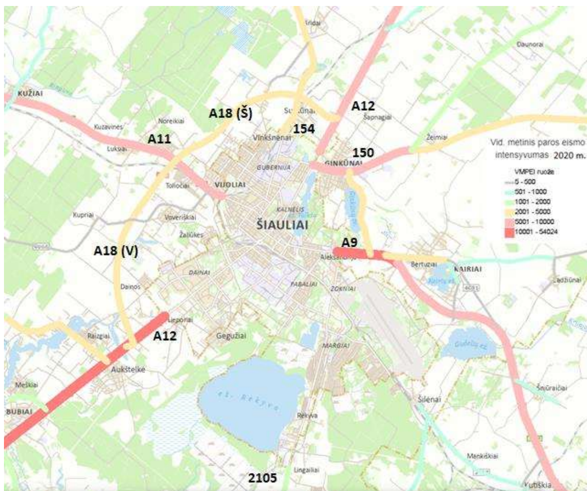
8 pav. Vidutinis metinis paros eismo intensyvumas magistraliniuose ir krašto keliuose Šiaulių miesto prieigose 2020 m.
