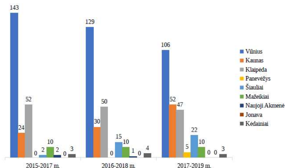
1 pav. Priešlaikinių mirčių, priskirtinų ilgalaikiam kietųjų dalelių poveikiui, skaičius Lietuvos miestuose 2015÷2019 m.
