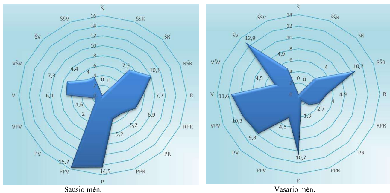
67 pav. Vėjo krypčių pasiskirstymas Šiauliuose 2021 m. sausio, vasario mėn.
