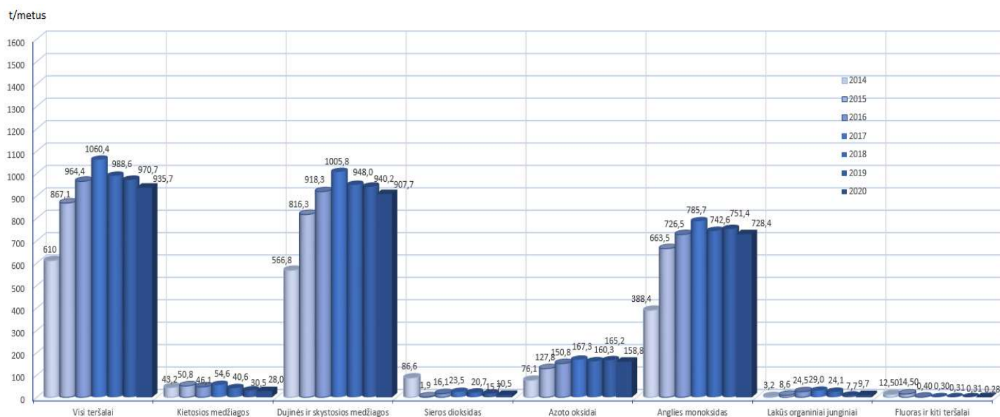
5 pav. Iš apskaitomų stacionarių aplinkos oro taršos šaltinių išmesto teršalų kiekio kitimas Šiauliuose 2014÷2020 m.
