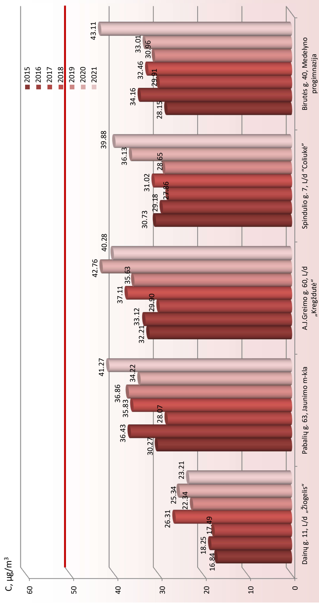
35 pav. Kietųjų dalelių ( \text{KD}_{10} ) vidutinės valandos koncentracijos kitimas lopšelių-darželių, mokyklų aplinkos ore 2015÷2021 m.
