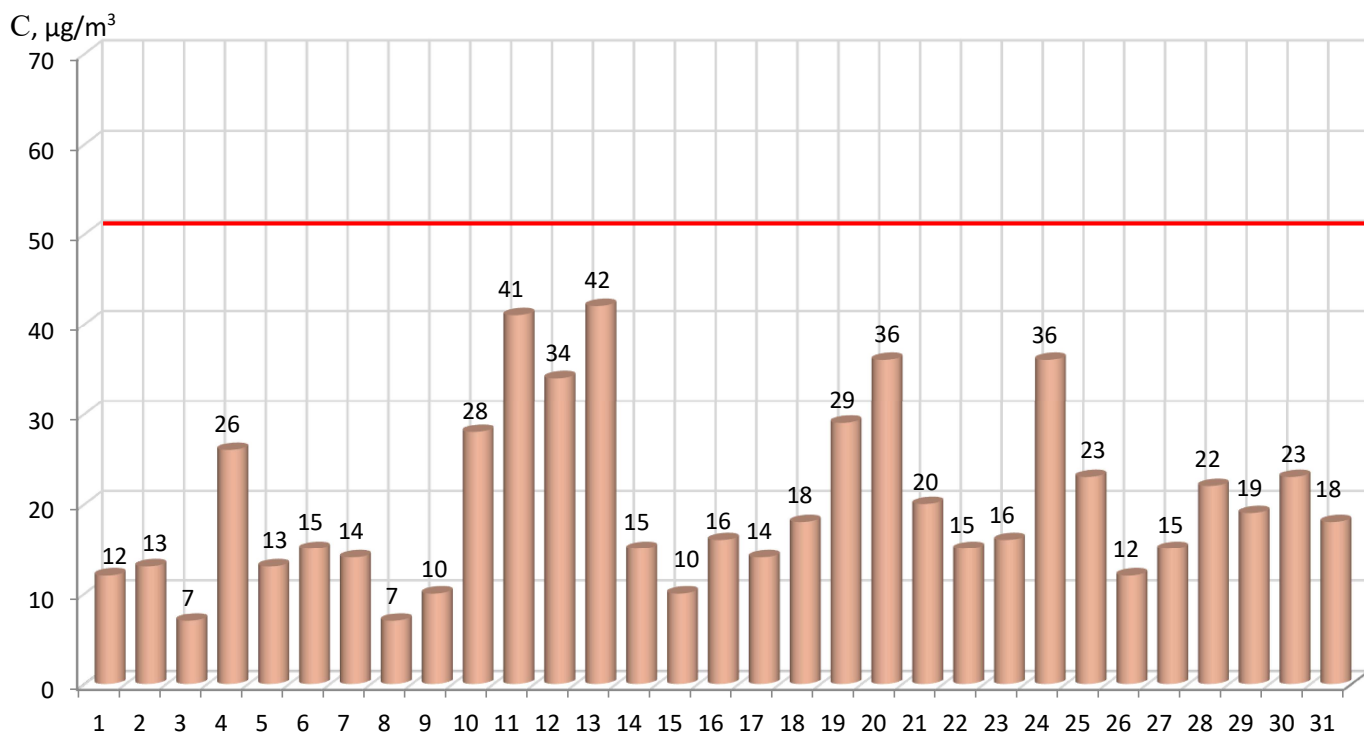
46 pav. Kietųjų dalelių ( \text{KD}_{10} ) vidutinės paros koncentracijos kitimas pietinėje miesto dalyje 2021 m. gegužės mėn. 1÷31 d.
