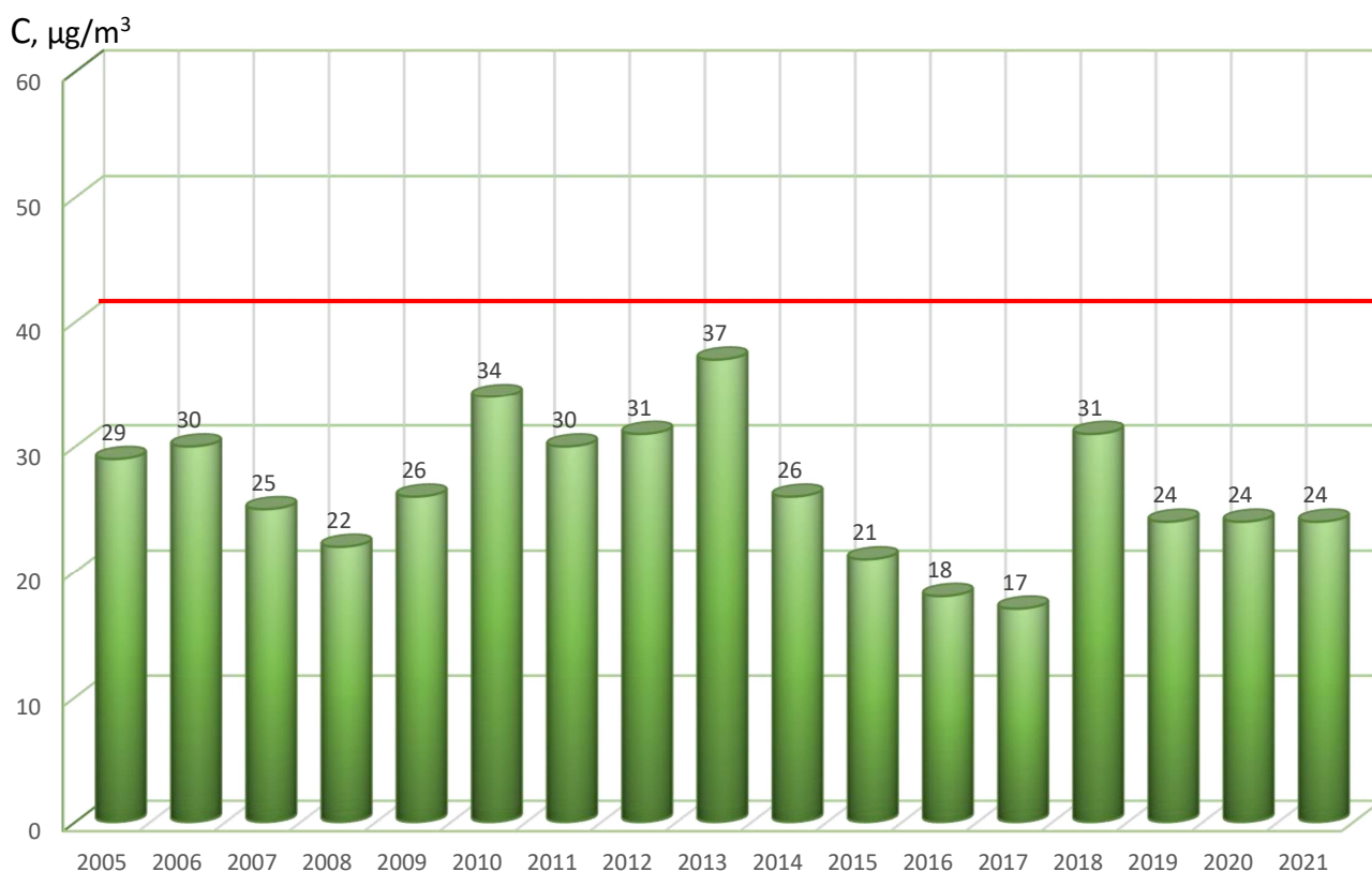
25 pav. Kietųjų dalelių (KD 10 ) vidutinės metų koncentracijos kitimas Šiauliuose 2005÷2021 m.
