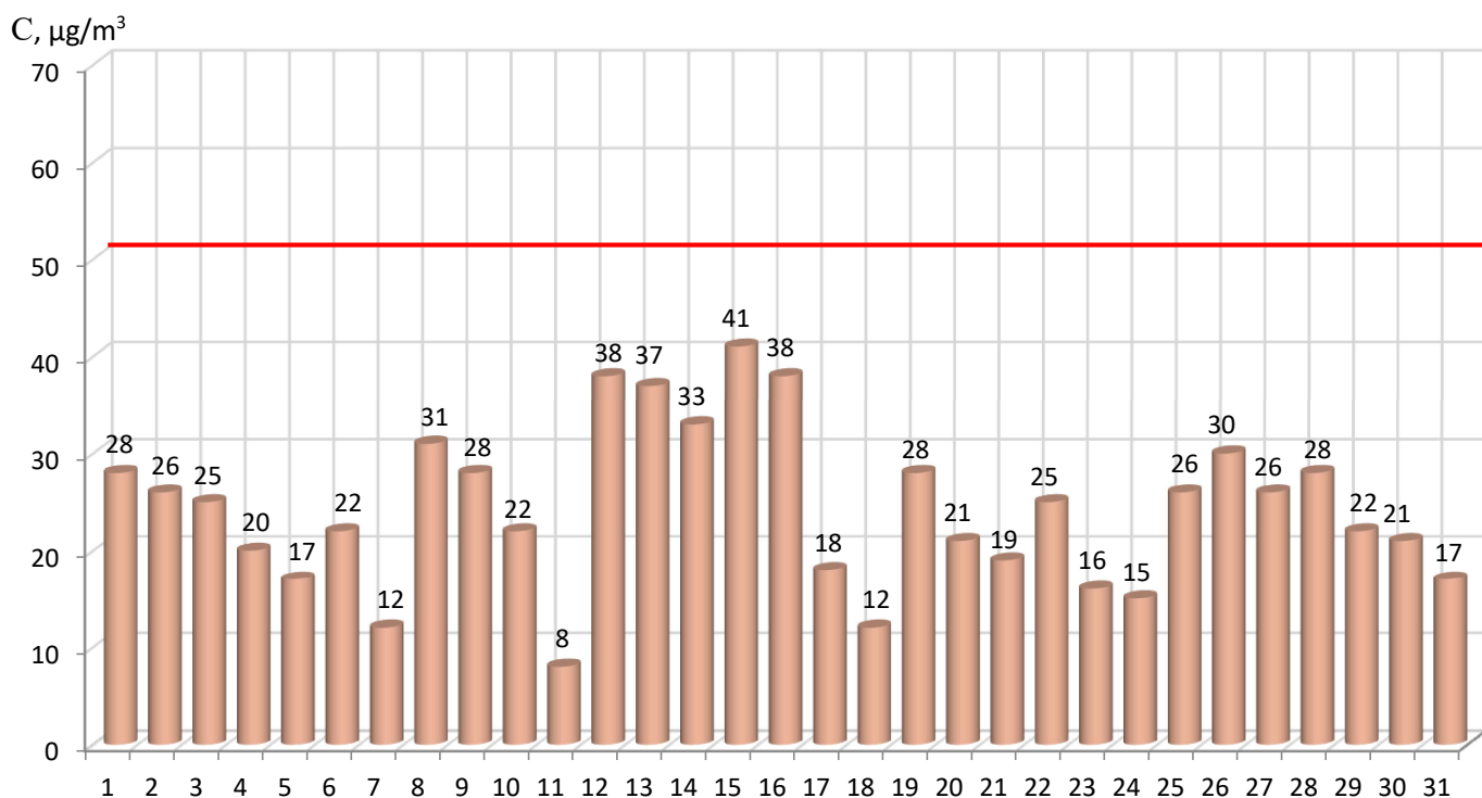
48 pav. Kietųjų dalelių ( \text{KD}_{10} ) vidutinės paros koncentracijos kitimas pietinėje miesto dalyje 2021 m. liepos mėn. 1÷31 d.
