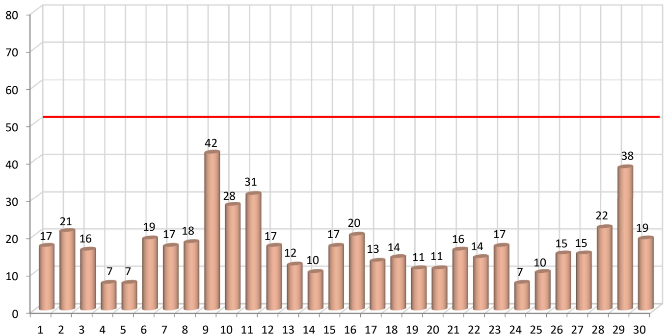
50 pav. Kietųjų dalelių ( \text{KD}_{10} ) vidutinės paros koncentracijos kitimas pietinėje miesto dalyje 2021 m. rugsėjo mėn. 1÷30 d.
